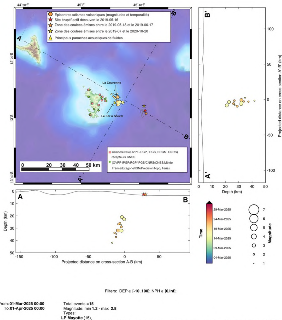
Figure 3 : Carte des épicentres ( \pm 5 km) des séismes longue période (LP) localisés avec les réseaux sismiques à terre (IPGP-CNRS-BRGM-BCSF-RENASS-ITES) en mars 2025 (échelle temporelle de couleur). Sont aussi représentées les projections des hypocentres des séismes le long de coupes transverses et axiales le long de la ride montrant la localisation estimée en profondeur (la précision varie entre \pm 5 km et \pm 15 km) des séismes en fonction de la magnitude (taille des symboles) et de la date (échelle temporelle de couleur). La localisation approximative des panaches acoustiques identifiés pendant les campagnes océanographiques est indiquée par des triangles jaunes, l'étoile rouge indique le site éruptif identifié le 16 mai 2019, l'étoile orange la zone des coulées émises entre le 18/05/2019 et le 17/06/2019 et l'étoile jaune la zone des coulées émises entre juillet 2019 et le 04/12/2020. Les structures volcaniques de la zone dites de « La Couronne » et du « Fer à Cheval » sont indiquées en grisé tout comme les coulées de lave de Fani Maoré. Les stations sismiques du réseau terrestre et les stations de positionnement par satellite GPS sont indiquées par des symboles (voir légende) (©OVPF-IPGP, BRGM, IFREMER, CNRS, BCSF-RENASS, ITES / REVOSIMA).
