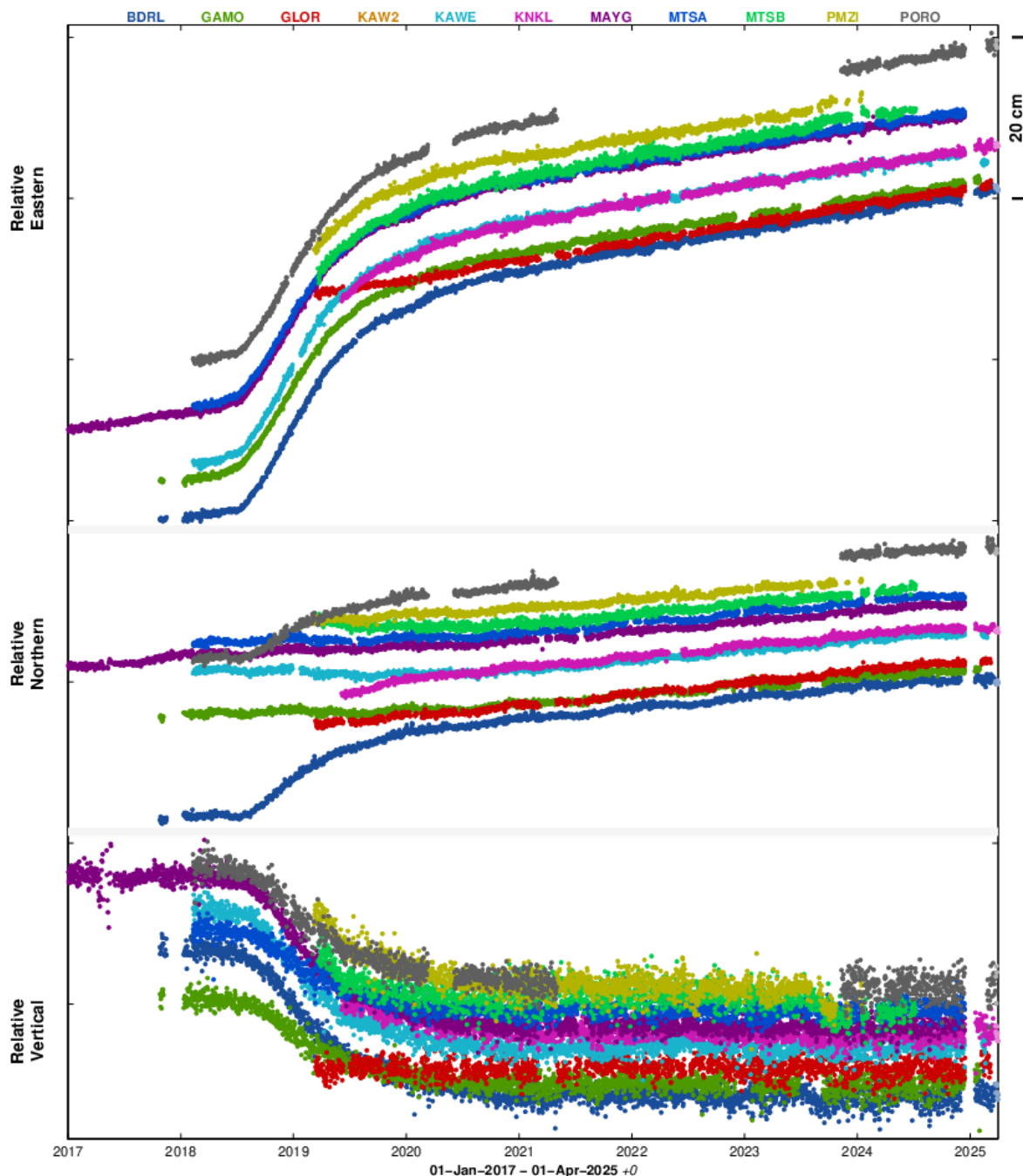
Figure 9 : Déplacements (en cm) enregistrés sur les stations GPS localisées à Mayotte (BDRL, GAMO, KAW1 remplacé en 2025 par KAW2, KNKL, MAYG, MTSA, MTSB, PMZI, PORO) et la station GLOR localisée à Grande Glorieuse sur les composantes est (en haut), nord (au milieu) et vertical (en bas) entre le 1 er janvier 2017 et 31 mars 2025 pour visualiser une longue série temporelle ante crise. Post-traitement de ces données réalisé par l'IPGP (©OVPF-IPGP / REVOSIMA). Suite au passage du cyclone Chido sur Mayotte le 14 décembre 2024, deux stations (MAYG et MTSA) ont été détruites, alors que les stations KNKL, KAW1, PORO, GAMO et BRDL ont subi des coupures électriques et/ou de transmission. En février 2025, une maintenance de la monumentation ainsi qu'un changement d'antenne à la station KAW1 ont conduit à la création d'une nouvelle station, KAW2 en remplacement de KAW1.
