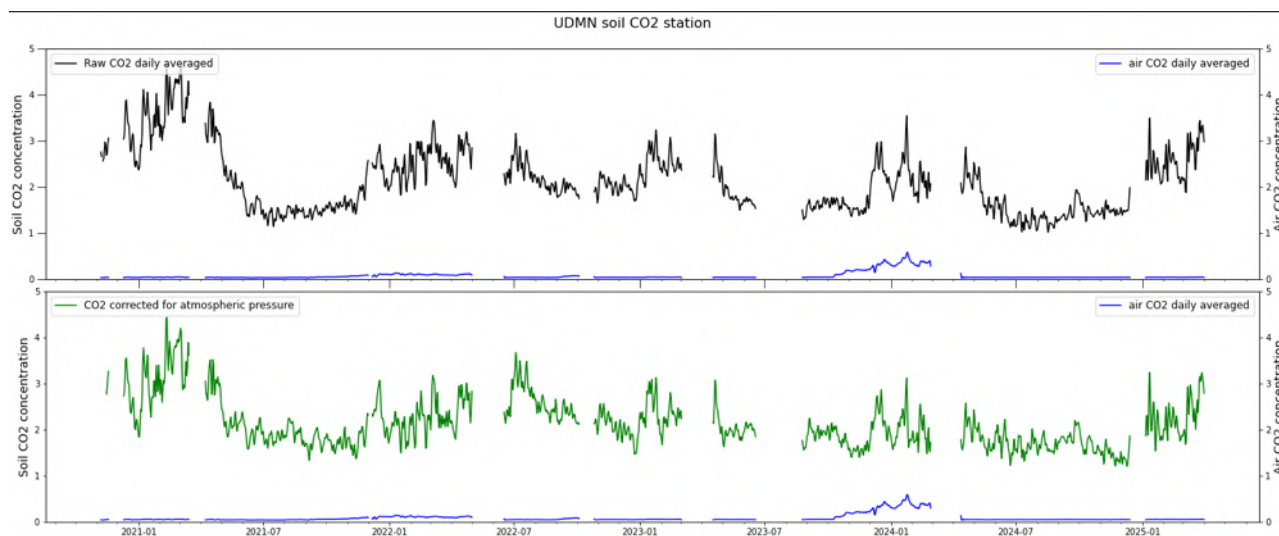
Figure 12 : Concentration en \text{CO}_2 dans le sol à la station permanente UDMN. Comparaison entre les données brutes (noir) et les données corrigées de l'influence de la pression atmosphérique (vert). Bleu : concentration du \text{CO}_2 dans l'air (1 m au-dessus du sol). Les variations de concentrations dans l'air sont liées à l'activité biogénique (©OVVPF-IPGP / REVOSIMA).
