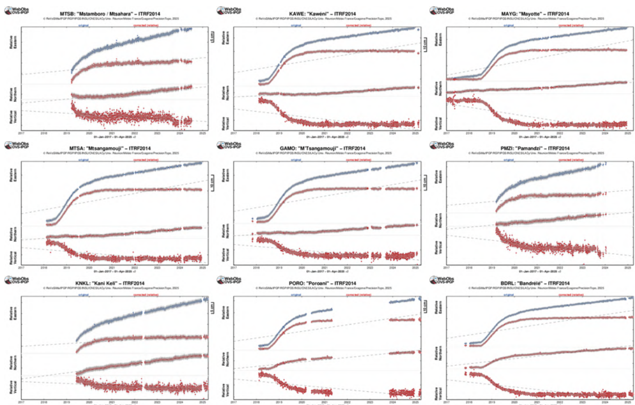
Figure 10 : Déplacements (en cm) enregistrés sur les stations GPS localisées à Mayotte (MTSB, KAWK, MAYG, MTSA, GAMO, PMZI, KNKL, PORO, BDRL) entre le 1 er janvier 2017 et le 31 mars 2025 pour visualiser une longue série temporelle ante crise. En bleu les données brutes, en rouge les données corrigées du mouvement de la plaque. Les stations sont présentées dans un ordre géographique ; du nord au sud (de haut en bas) et d'ouest en est (de gauche à droite). Post-traitement de ces données réalisé par l'IPGP (©OVPF-IPGP / REVOSIMA). Suite au passage du cyclone Chido sur Mayotte le 14 décembre 2024, deux stations (MAYG et MTSA) ont été détruites, alors que les stations KNKL, KAWK, PORO, GAMO et BDRL ont subi des coupures électriques et/ou de transmission. En février 2025, une maintenance de la monumentation ainsi qu'un changement d'antenne à la station KAWK ont conduit à la création d'une nouvelle station, KAW2 en remplacement de KAWK.
