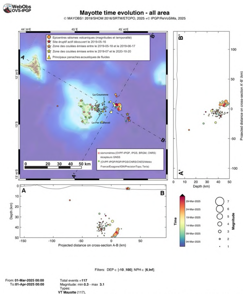
Figure 2 : Carte des épicentres ( \pm 5 km) des séismes volcano-tectoniques (VT) localisés avec les réseaux sismiques à terre (IPGP-CNRS-BRGM-BCSF-RENASS-ITES) en mars 2025 (échelle temporelle de couleur). Sont aussi représentées les projections des hypocentres des séismes le long de coupes transverses et axiales le long de la ride montrant la localisation estimée en profondeur (la précision varie entre \pm 5 km et \pm 15 km) des séismes en fonction de la magnitude (taille des symboles) et de la date (échelle temporelle de couleur). La localisation approximative des panaches acoustiques identifiés pendant les campagnes océanographiques est indiquée par des triangles jaunes, l'étoile rouge indique le site éruptif identifié le 16 mai 2019, l'étoile orange la zone des coulées émises entre le 18/05/2019 et le 17/06/2019 et l'étoile jaune la zone des coulées émises entre juillet 2019 et le 04/12/2020. Les structures volcaniques de la zone dites de « La Couronne » et du « Fer à Cheval » sont indiquées en grisé tout comme les coulées de lave de Fani Maoré. Les stations sismiques du réseau terrestre et les stations de positionnement par satellite GPS sont indiquées par des symboles (voir légende) (©OVPF-IPGP, BRGM, IFREMER, CNRS, BCSF-RENASS, ITES / REVOSIMA).
