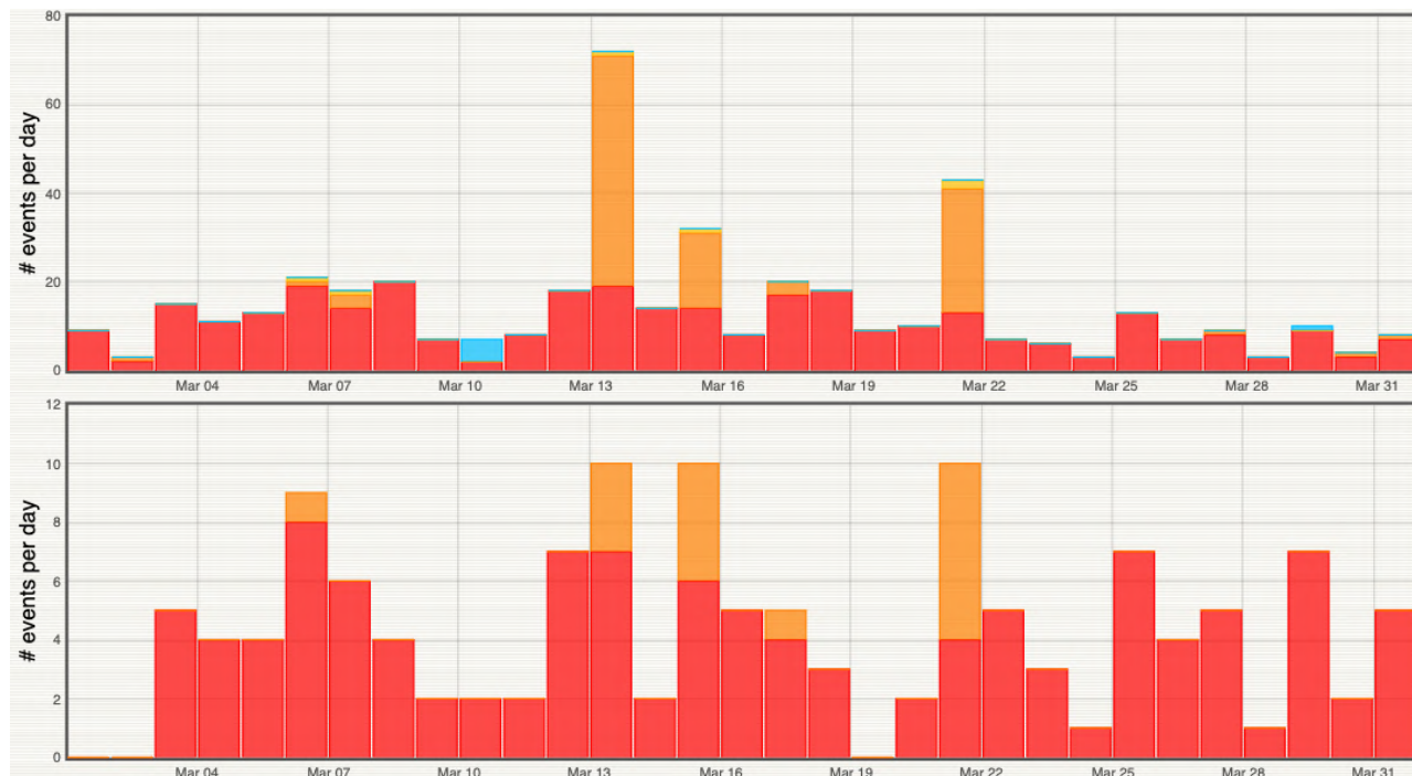
Figure 7 : Histogramme représentant le nombre de séismes par jour détectés (en haut) et localisés (en bas) en mars 2025 par le réseau sismologique du REVOSIMA. En rouge les séismes volcano-tectoniques, en orange les séismes longues périodes, en jaune les séismes très longues périodes, en bleu les ondes sonores liées aux orages (© OVPF-IPGP et REVOSIMA).
